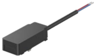
Tracc-ACC-BCB-NG Accesorio de conexión para entrada de voltaje para tracklight en color negro
